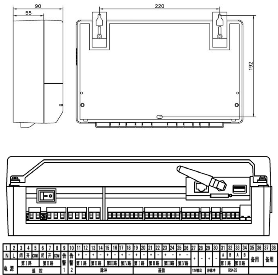
图 1 接线端子示意图
