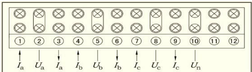
图 3 电源端子接线图
