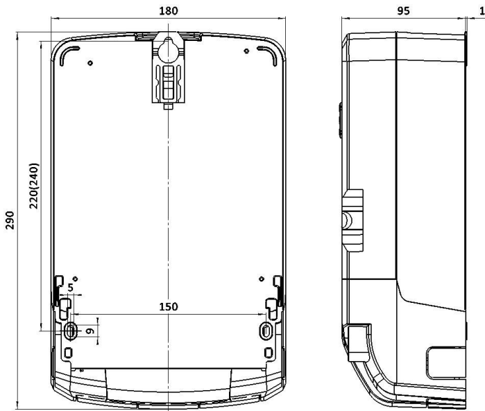
图 1 终端外形及安装尺寸图
